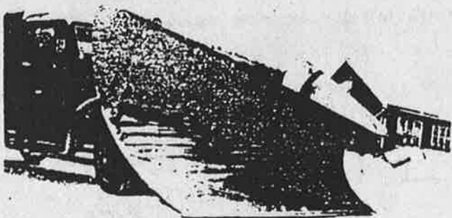
Fig. 202. Stor forplog fra Møre og Romsdal fylke. Plogarmene er festet med en bolt på midten og regulerbare foran.
