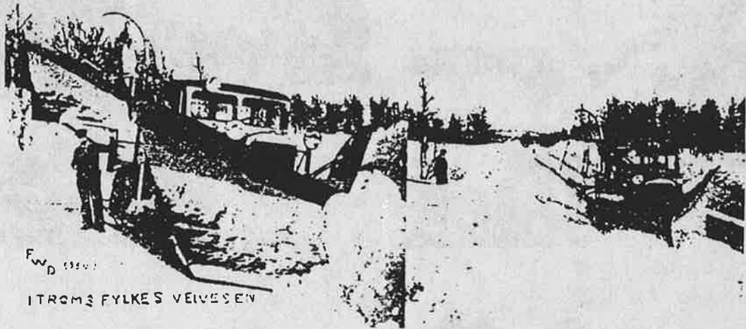
Fig. 212. Forplog og kantplog. Vegvesenet i Troms fylke. Kantploegen henger i en david.
