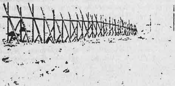
Fig. 231. Skjelett til fast snøskjerm på Hardangervidda.
