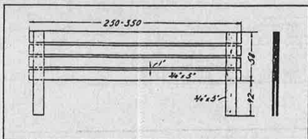
Fig. 227. «Rytter» til forhøyelse av nedfokne snøskjermer. (Mål i cm.)
