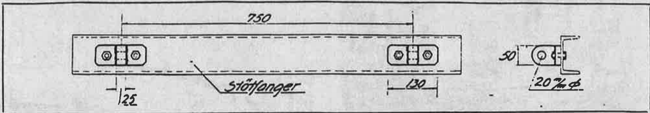
Fig. 201. Plogfeste på støttfangeren. (Mål i mm.)
