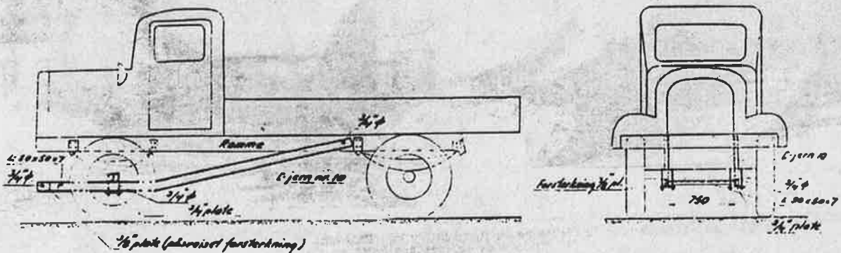
Fig. 206. Plogfeste som overfører kraften til rammen ved bilens bakhjul. Armene som lett kan tas vekk om sommeren settes av vinkeljern eller kanaljern.
