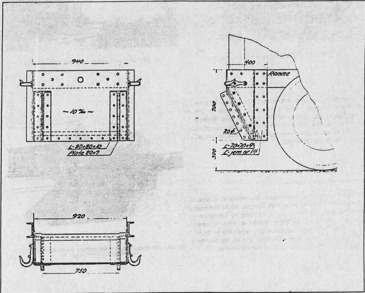
Fig. 205. Solid plogfeste på bilrammen — er alminnelig brukt på F. W. D. brytebiler. (Mål i mm.)
