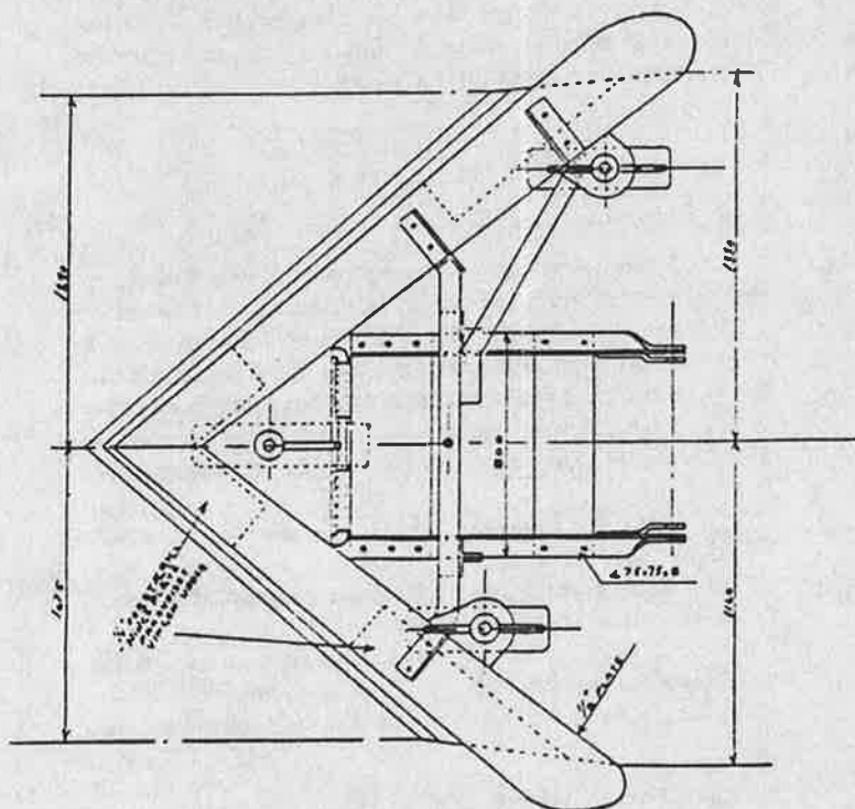
Fig. 198. Ankerløkkens forplog nr. 3 med forlenget høyreving.
