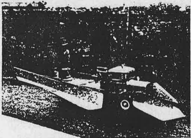
Fig. 211. Forplog og sideplog. Vegvesenet i Sør-Trøndelag fylke. Sideplogen manøvreres av en mann som sitter på lasteplatten. Plogen er opprinnelig uteksperimentert ved Seiburuten for vegvesenets midler og er senere delvis omkonstruert ved vegvesenets verksted.
