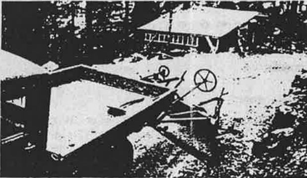
Fig. 220. En bakplog fra Rogaland for å fjerne snøplogkanten langs fjellvegg.
