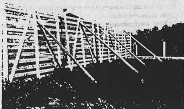
Fig. 228. Flyttbar snøskjerm fra Dovre—Hjerkin. Avstivet med strevere og barduner til begge sider.
