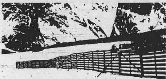
Fig. 228. Flyttbar snøskjerm fra Dovre—Hjerkin. Avstivet med strevere og barduner til begge sider.
