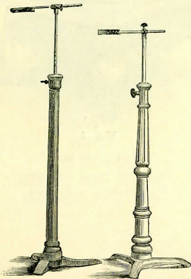
Nackhållare för fotografer.
