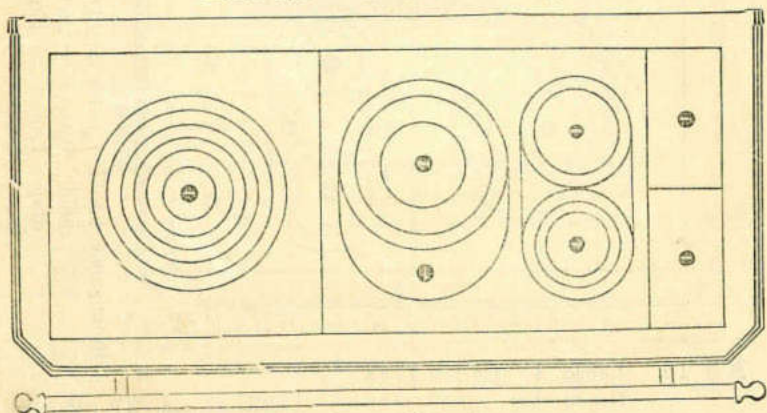
N:o 18. Längd 5 fot = 1485 m/m Bredd 2,50 > = 742 > Pris, se sid. 27.
