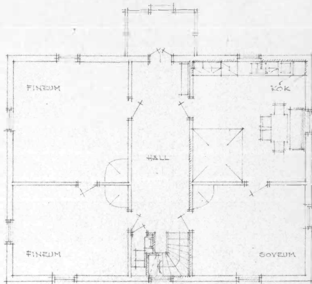
BOTTENVÅNING
