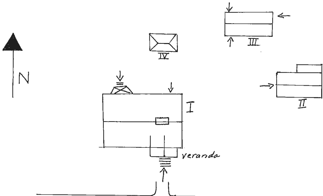
Situationsplan Älven
