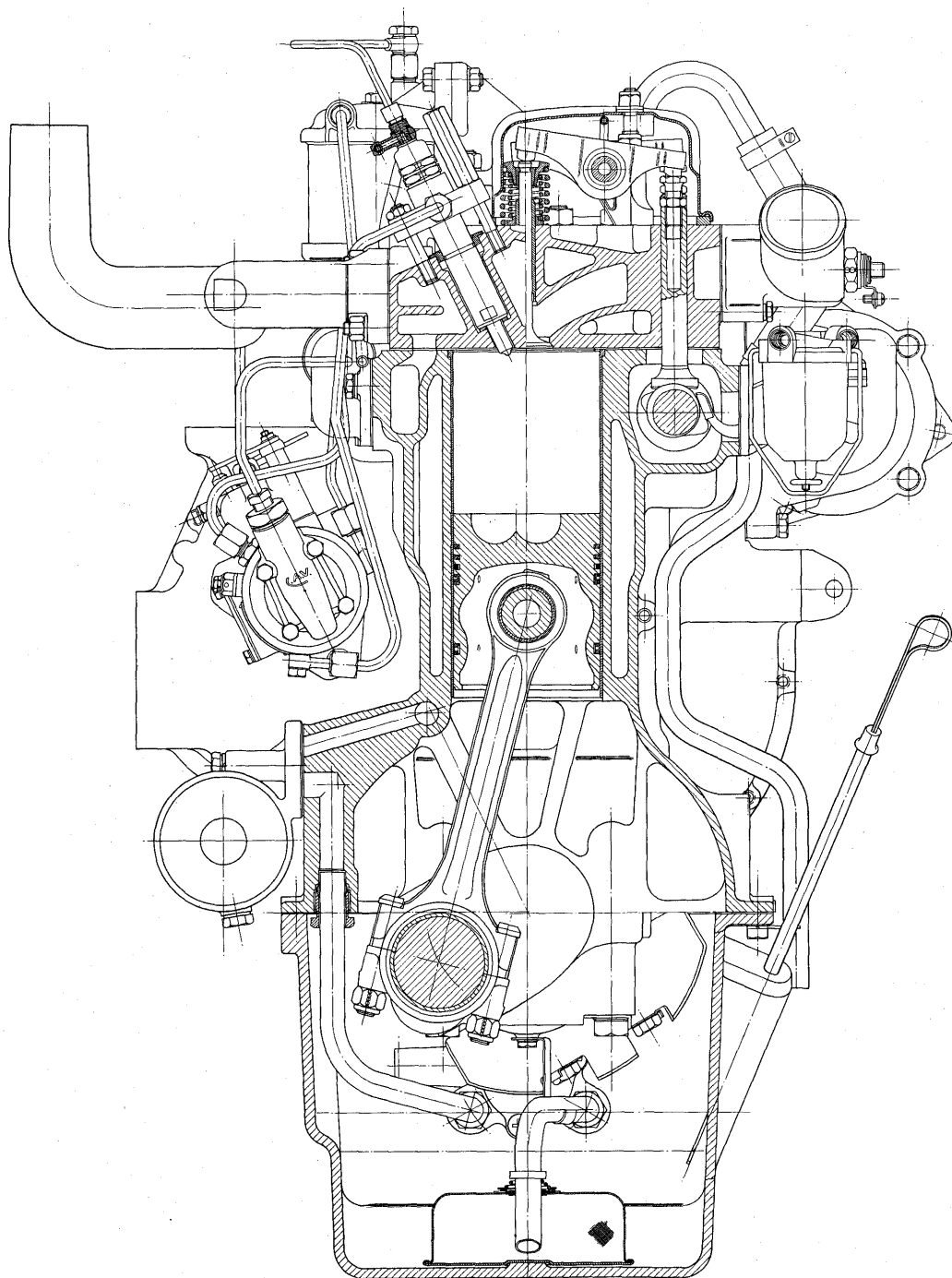
Fig. 20. Tværsnit motor.
