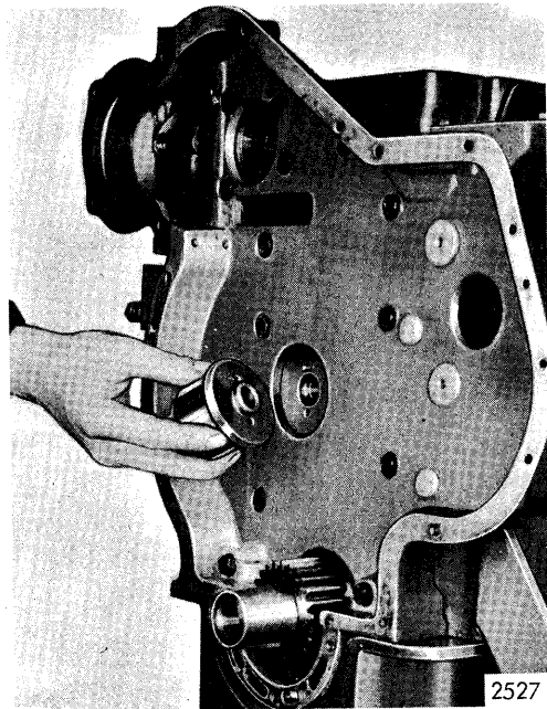
Fig. 10. Mellemdrevets lejetap.
