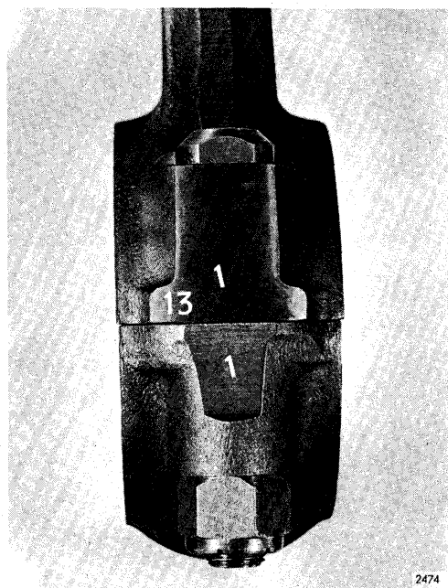
Fig. 6. Plejlstængernes mærkning.
