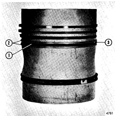
Fig. 4. Stempelringsmonteringen.
