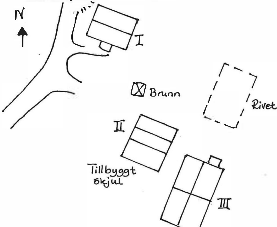
Situationsplan Jordkällare
